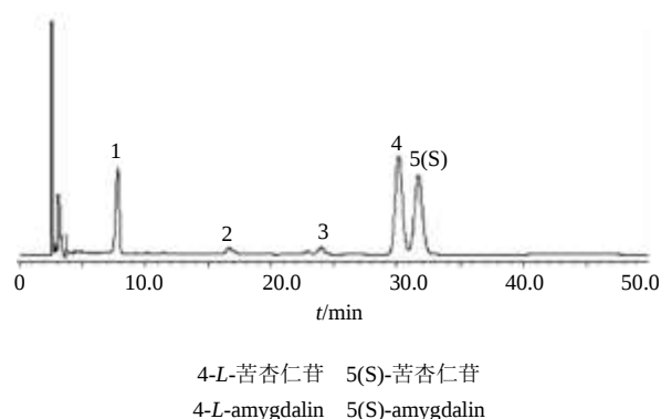
图 3 燀苦杏仁配方颗粒特征图谱
