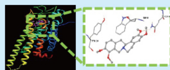
分子对接
