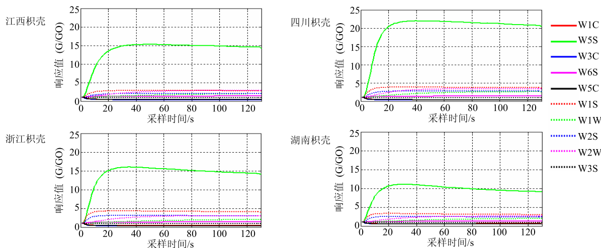
图 1 不同产地枳壳气味采集响应曲线
