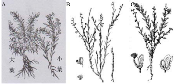
A-《纲目》大叶、小叶远志 B-《中华本草》远志 C-《中华本草》卵叶远志
