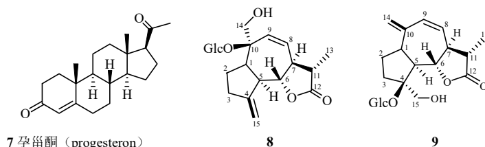
图 3 化合物 7~9 的化学结构
