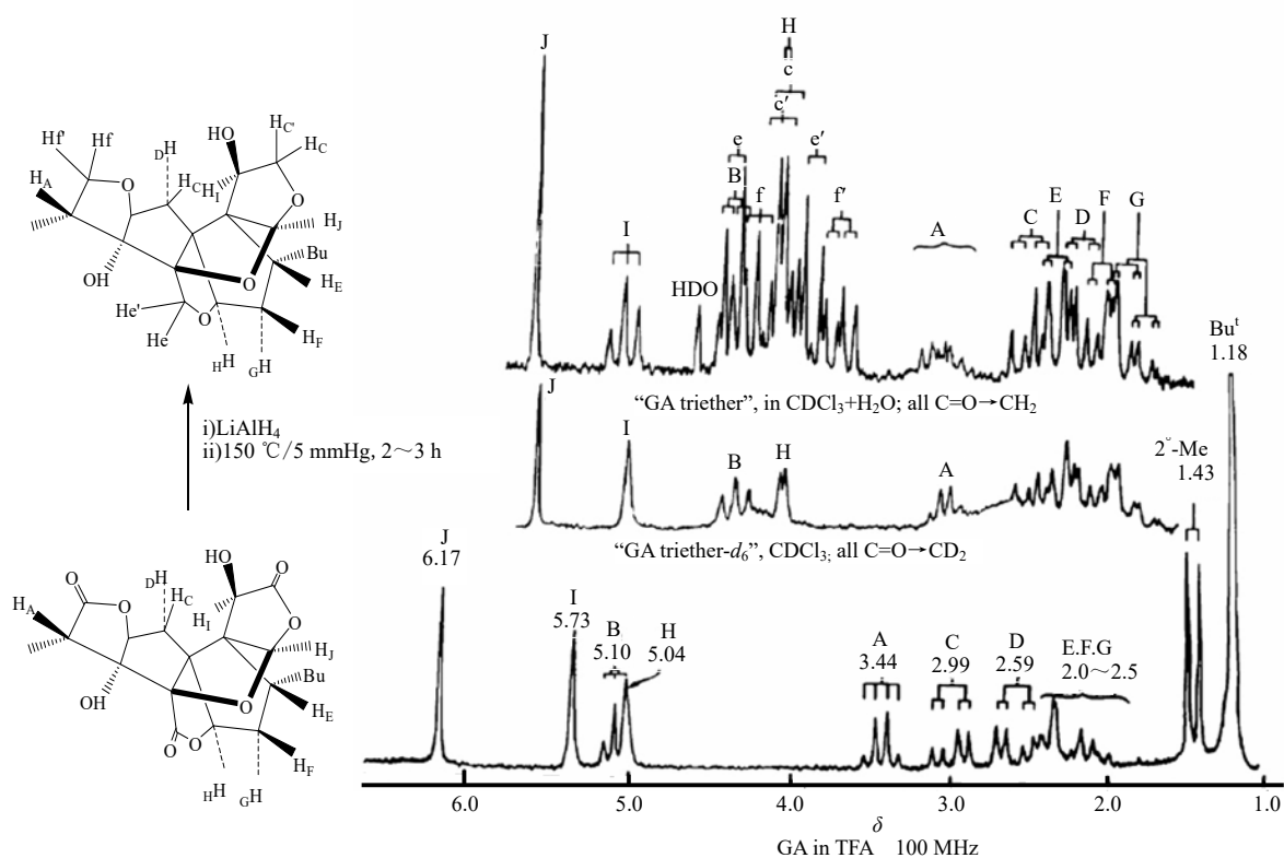
图 12 银杏内酯 (18) 的化学结构及其 ^1\text{H} -NMR 谱
