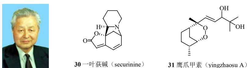
图 20 梁晓天院士以及一叶荻碱、鹰爪甲素的化学结构
