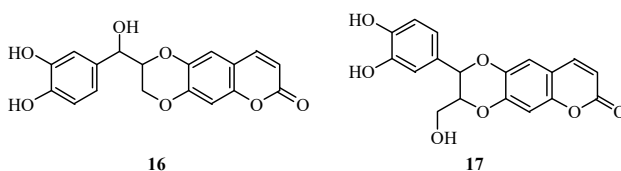
图 9 化合物 16 和 17 的化学结构
