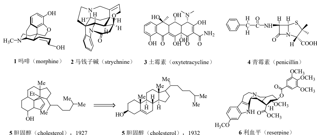
图 1 具有历史意义的部分天然产物的化学结构
