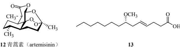
图 6 青蒿素和化合物 13 的化学结构
