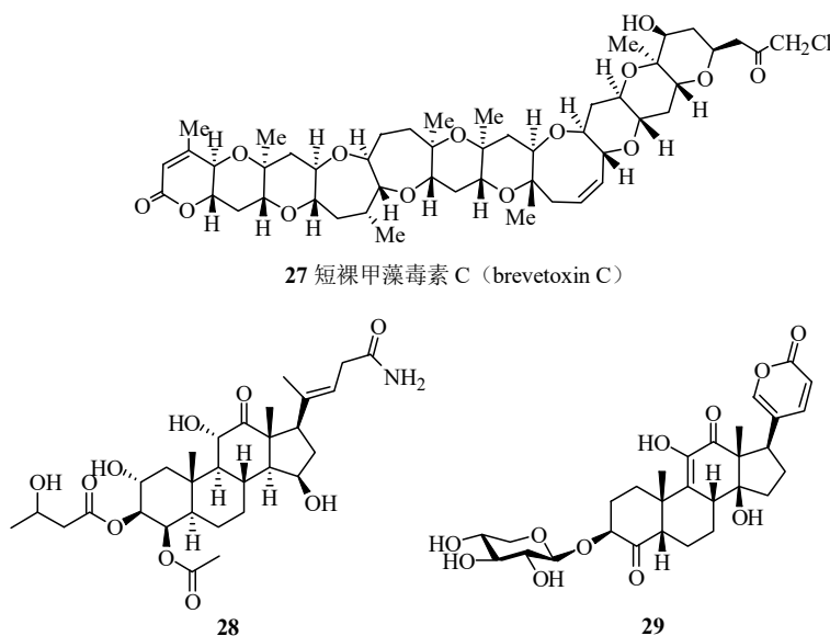
图 19 Brevetoxin C 以及化合物 28 和 29 的化学结构
