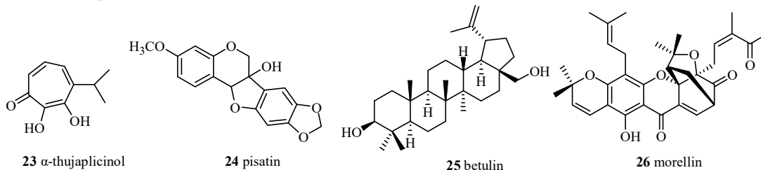
图 15 化合物 23~26 的化学结构
