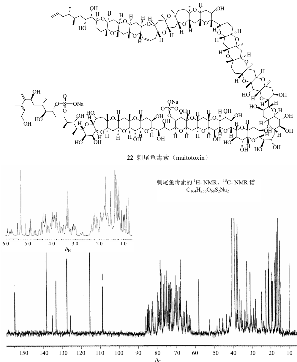
图 14 刺尾鱼毒素的化学结构及其 ^1H -NMR、 ^{13}C -NMR 谱
