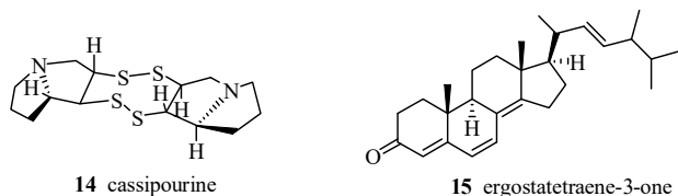
图 7 化合物 14 和 15 的结构
