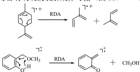
图 10 RDA 裂解
