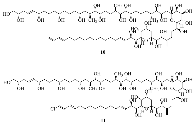
图 4 化合物 10、11 的化学结构
