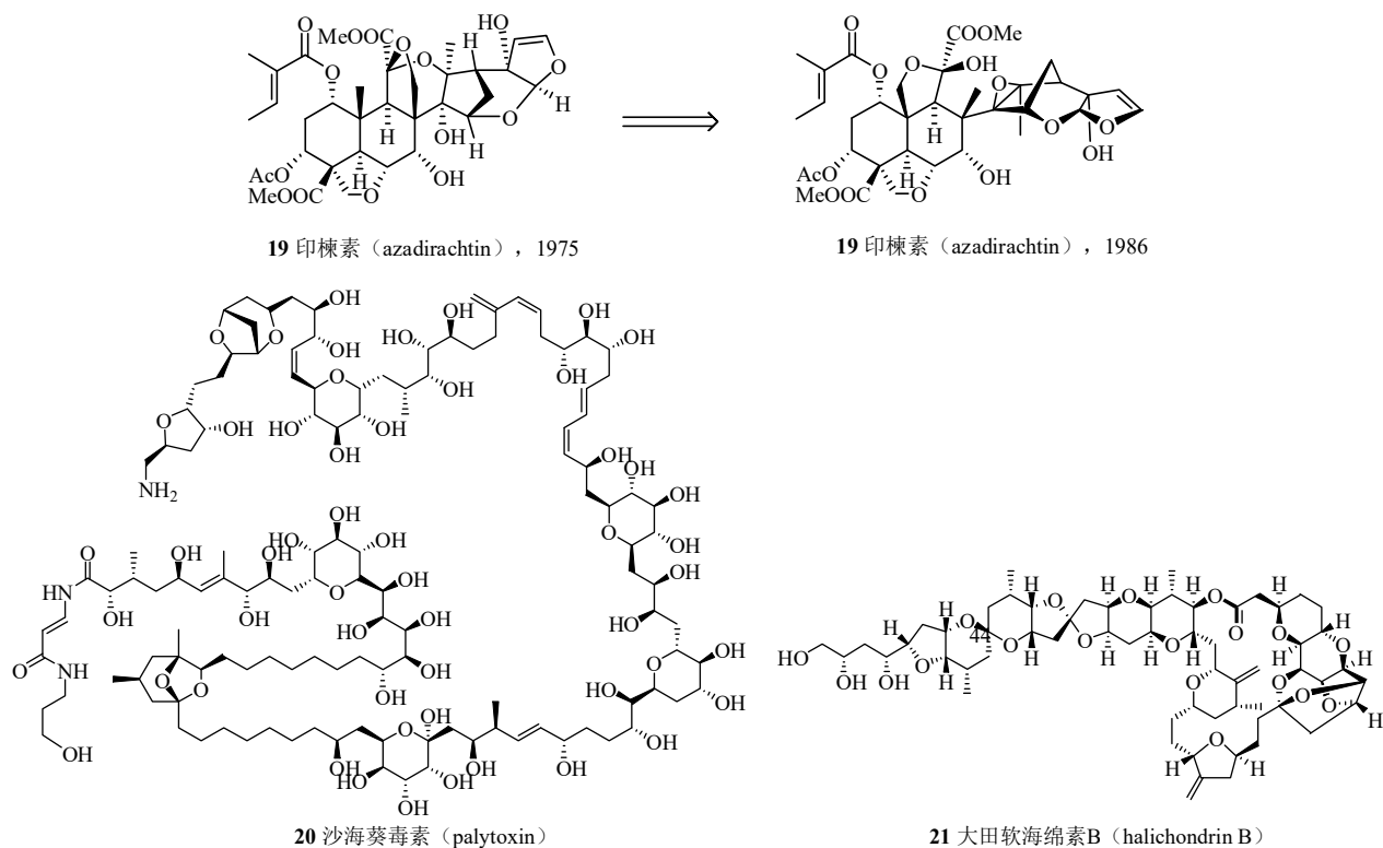
图 13 化合物 19~21 的化学结构
