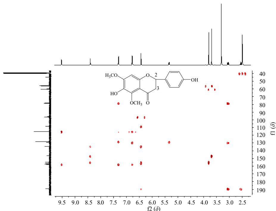
图 16 一个黄酮的化学结构及其 HMBC 谱
