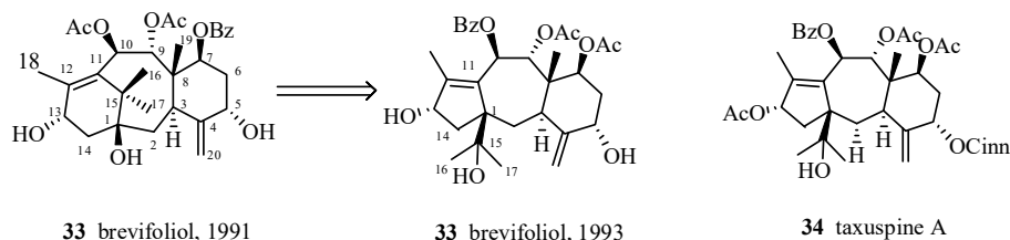
图 22 化合物 33 和 34 的化学结构
