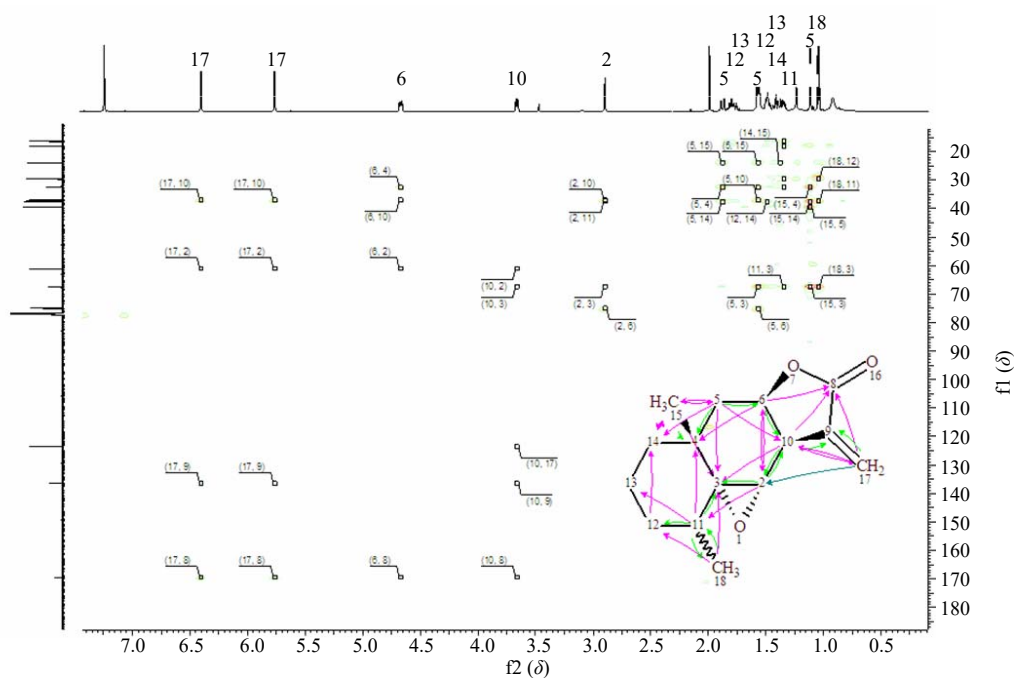
图 17 一个倍半萜的化学结构及其 HMBC 谱
