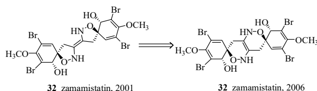
图 21 Zamamistatin 的化学结构
