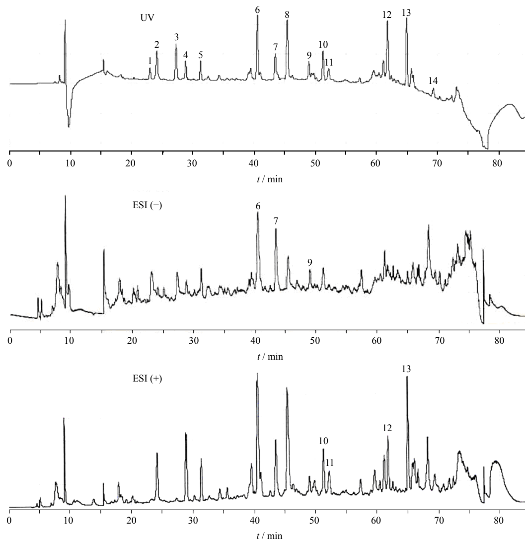
图 2 强肝胶囊样品液质图谱
