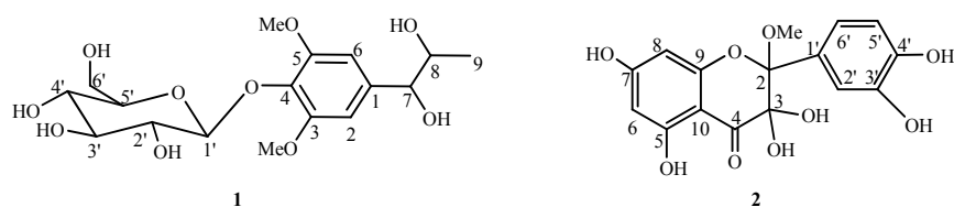
图 1 化合物 1 和 2 的结构
