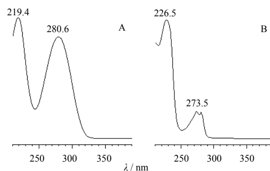
图 3 洋川芎内酯 A (A) 和新化合物 (B) 的紫外光谱图 Fig. 3 UV spectra of senkyunolide A (A) and new compound (B)
