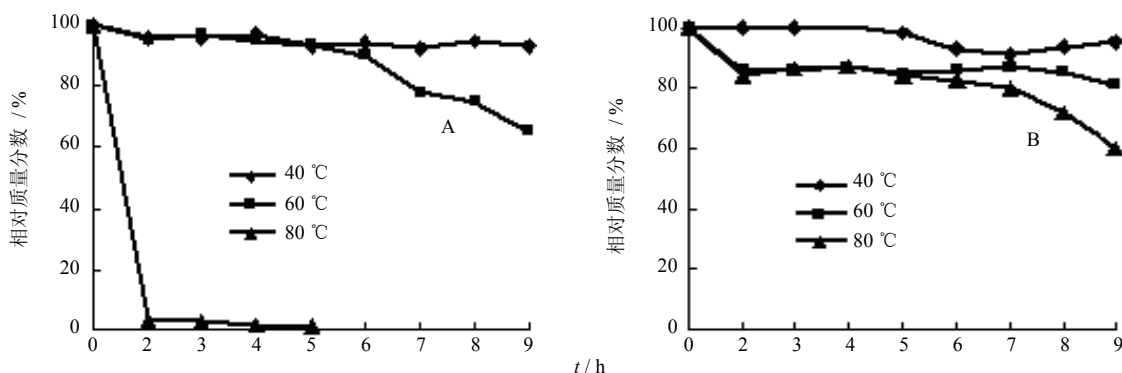
图 1 洋川芎内酯 A (A) 和洋川芎内酯 I (B) 不同温度、时间质量分数变化
