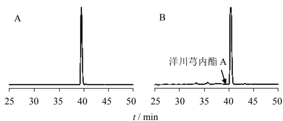
图 2 洋川芎内酯 A (A) 及其室温自然光照 2 个月后的样品 (B) 的 HPLC 图
