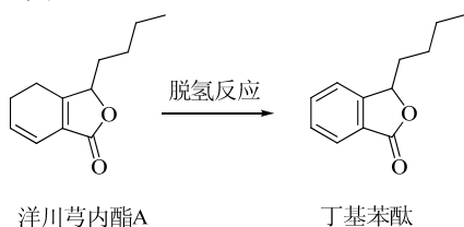
图 5 洋川芎内酯 A 的降解途径
