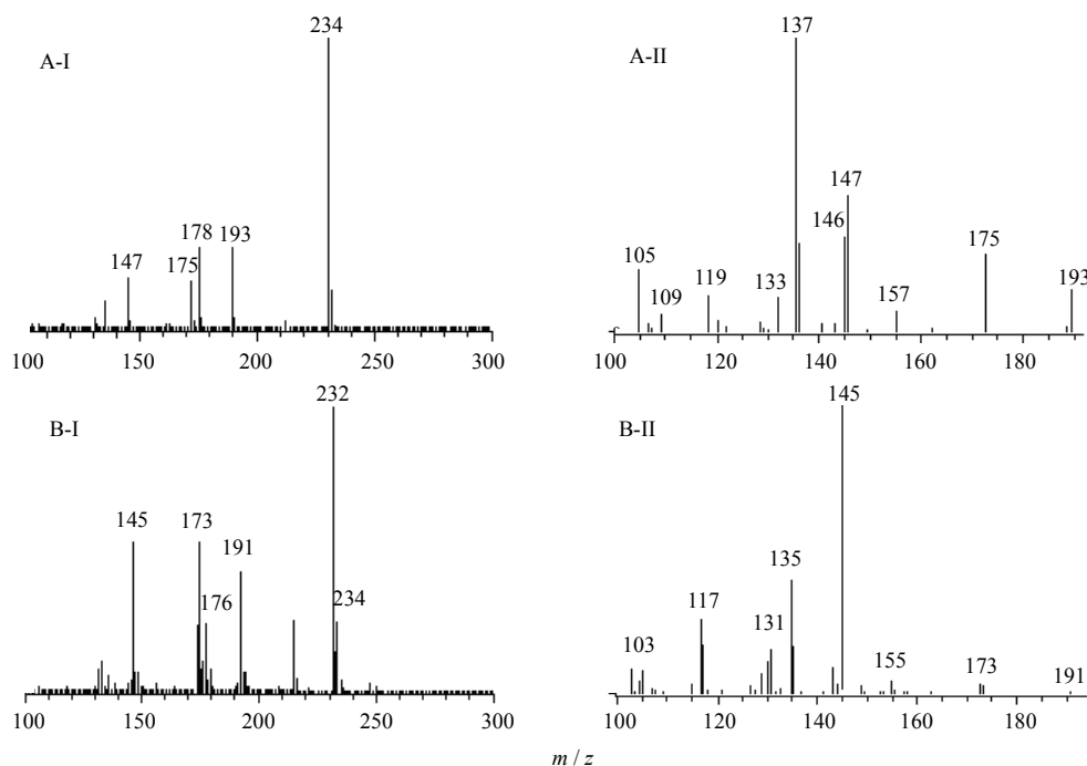
图 4 洋川芎内酯 A (A) 和新化合物 (B) 的一级 (I)、二级 (II) 质谱图 Fig. 4 MS (I) and MS 2 (II) spectra of senkyunolide A (A) and new compound (B)
