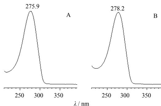
图 7 洋川芎内酯 I (A) 和新化合物 (B) 紫外光谱图
