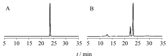
图 6 洋川芎内酯 I (A) 及其室温自然光照 2 个月后的样品 (B) 的 HPLC 图
