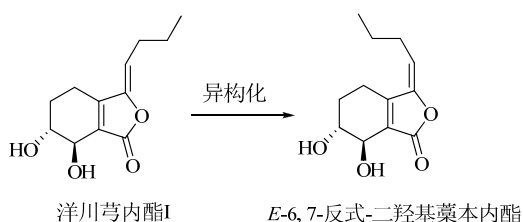
图8 洋川芎内酯 I 的降解途径 Fig. 8 Degradation pathway of senkyunolide I
