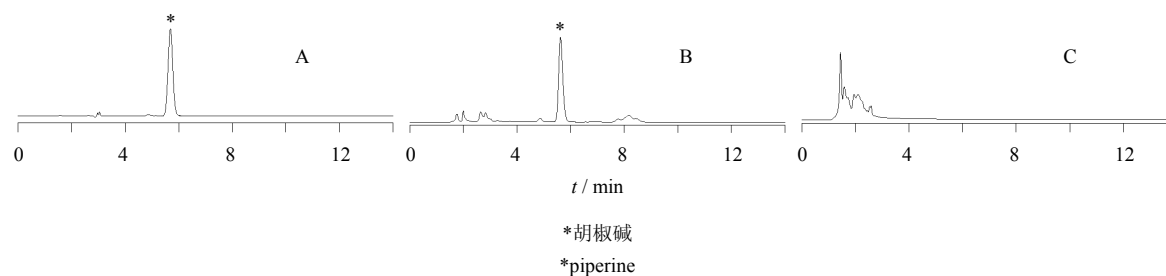
图 2 胡椒碱对照品 (A)、镇痛灵方合煎样品 (B)、阴性样品 (C) 的 HPLC 图 Fig. 2 HPLC chromatograms of piperine reference substance (A), combined decoction of ZTLP sample (B), and negative sample (C)
