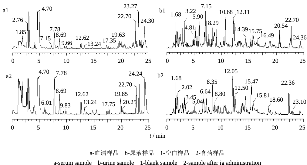
图4 血清样品和尿液样品正离子流色谱图
