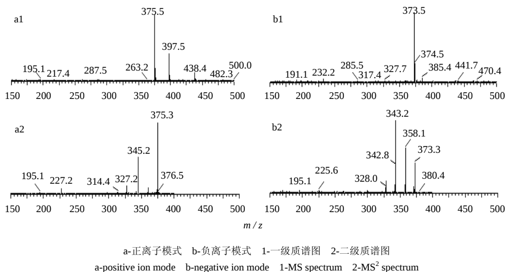
图 2 黄芩新素 II 的一级和二级质谱图
