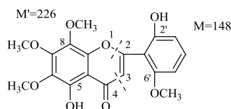
图 3 黄芩新素 II 结构式
