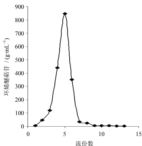
图 2 梔子环烯醚萜苷在 D-101 大孔吸附树脂上的洗脱曲线
