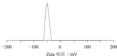
图 4 表面电位图
