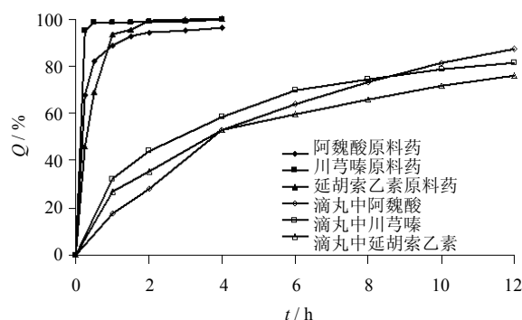
图 2 内异消复方缓释滴丸和原料药的体外释药曲线 ( n=3 )
