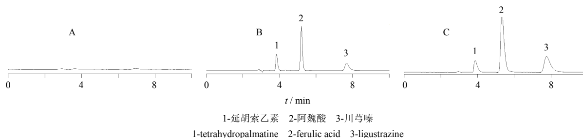
图 1 空白滴丸 (A)、混合对照品溶液 (B) 和样品溶液 (C) 的 HPLC 图
