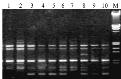
图 2 10 批白头翁 OpeE 16 引物不同模板 DNA 扩增产物图谱
