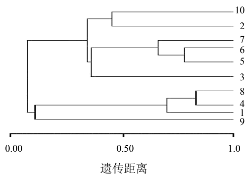
图 3 10 个不同基因型的白头翁 DNA 多态性聚类分析树型图
