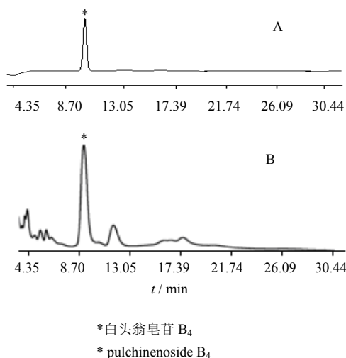
图 6 对照品 (A) 与样品 (B) 的 HPLC 图
