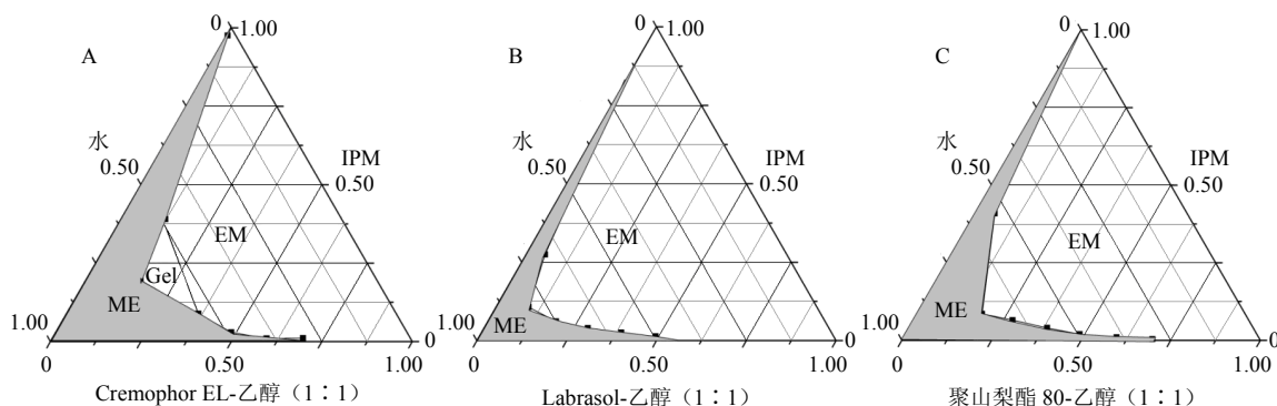
图 3 不同的表面活性剂 Cremophor EL (A)、Labrasol (B) 和聚山梨酯 80 (C) 组成微乳的伪三元相图
