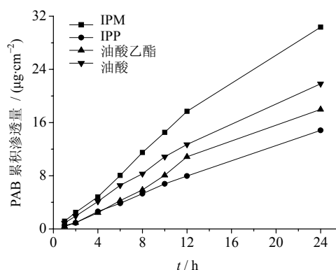
图 2 PAB 在不同油相组成的微乳中的体外经皮渗透曲线 ( \bar{x} \pm s , n=3 )
