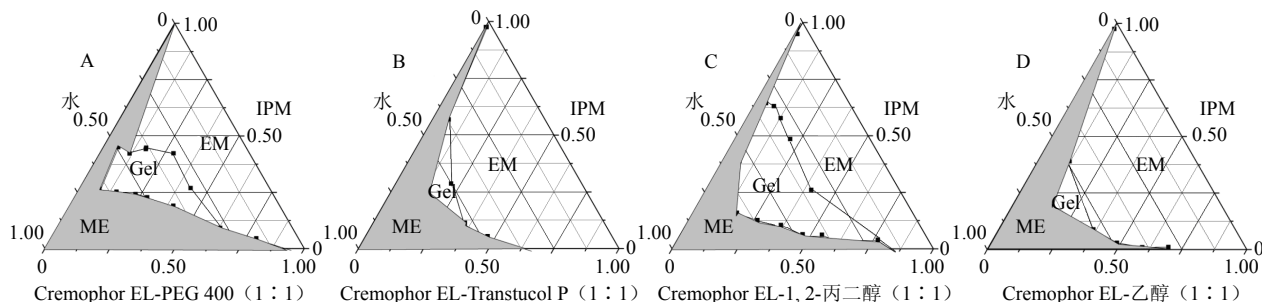
图 4 不同的助表面活性剂 PEG 400 (A)、Transcutol P (B)、1,2-丙二醇 (C)、乙醇 (D) 组成微乳的伪三元相图
