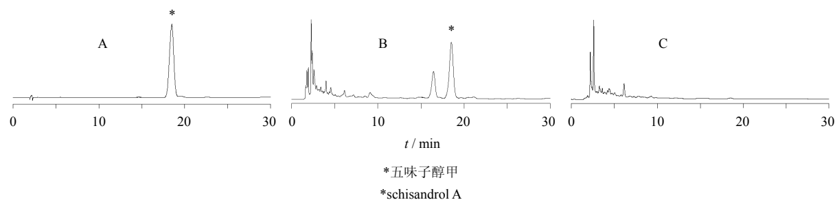
图1 对照品(A)、参芪五味子分散片(B)和阴性样品(C)的HPLC图
