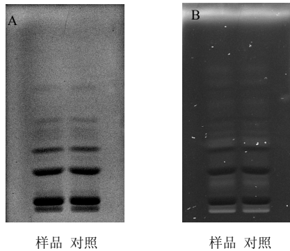
图 1 日光 (A) 和紫外光灯 (B) 下西红花的薄层色谱图 Fig. 1 TLC chromatograms of C. sativus in sunlight (A) and UV light (B)
