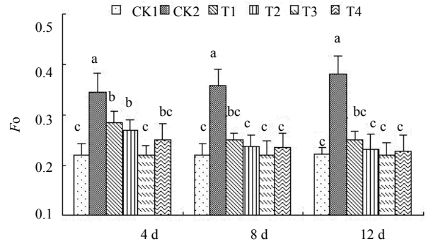
图 5 F_o 的变化
