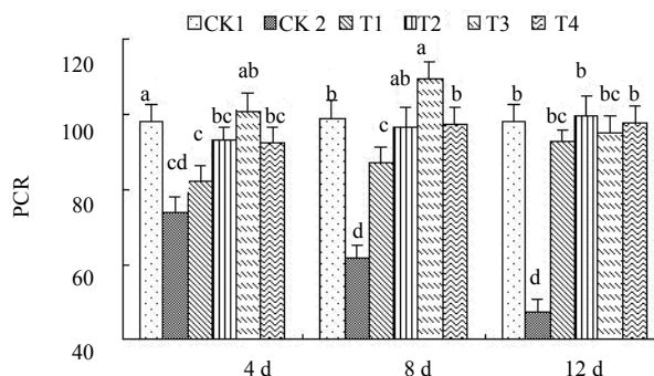
图 15 PCR 的变化
