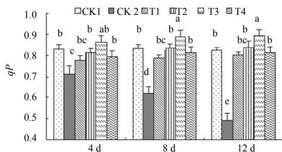
图 11 qP 的变化
