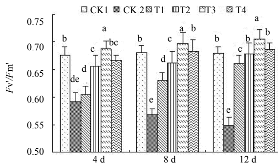
图9 F_v/F_m' 的变化
