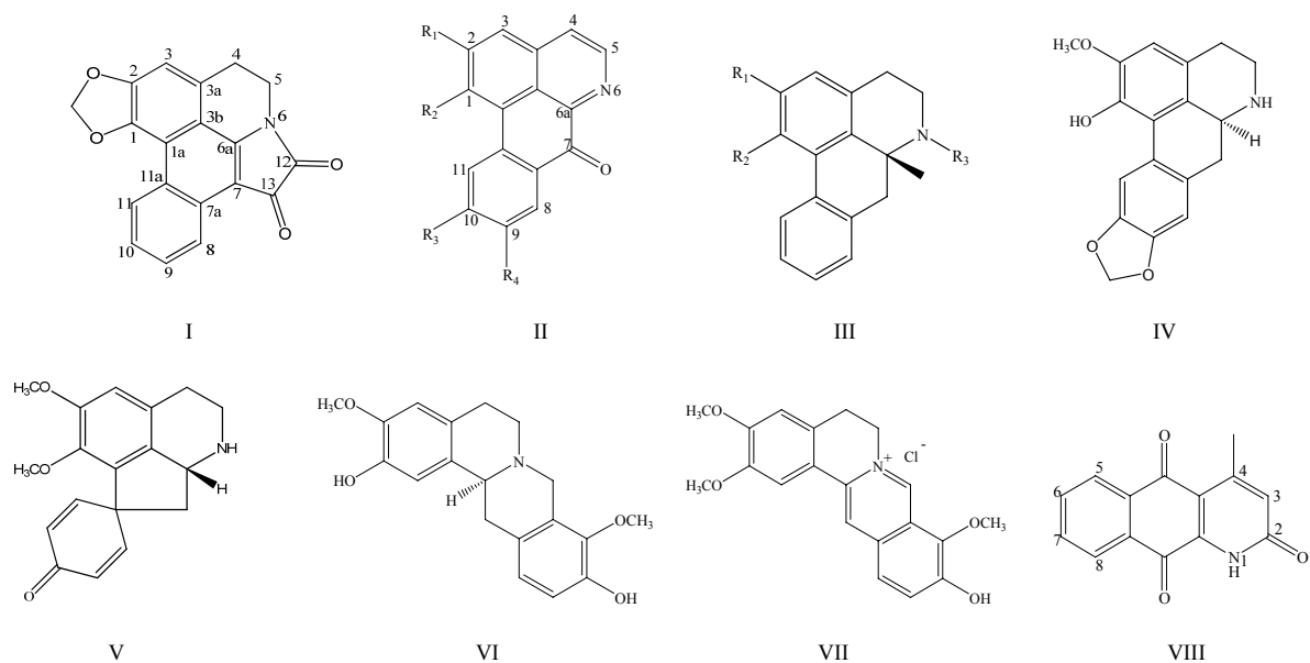
图4 圆滑番荔枝植物中生物碱类化合物的类型 Fig. 4 Types of alkaloid compounds in A. glabra
