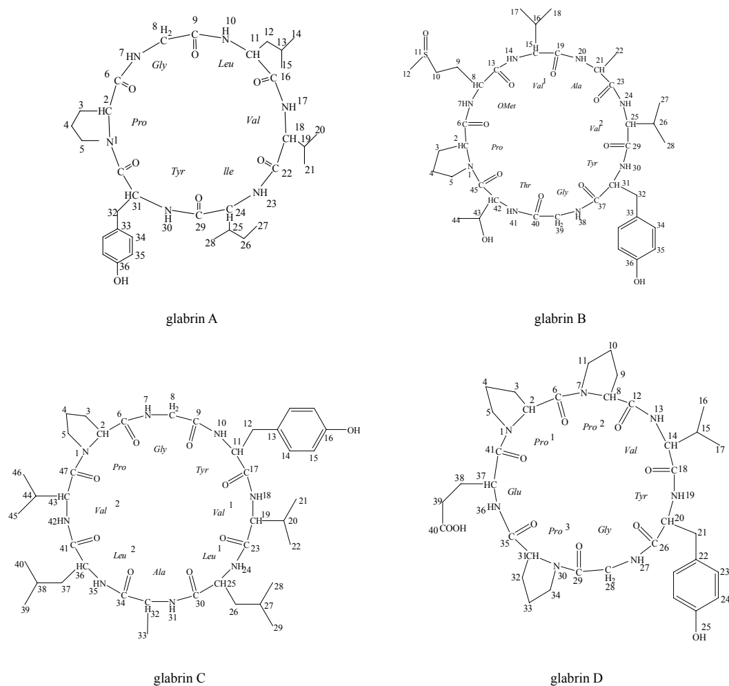
图3 圆滑番荔枝植物中环肽类化合物 Fig. 3 Cyclopeptide compounds in A. glabra
