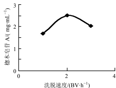
图6 洗脱速度对橐木皂苷A的影响 Fig. 6 Effect of eluting velocity on araloside A
