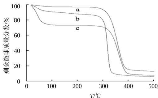
图 3 \beta -CD (a)、 \beta -CDP 微球 (b) 及薄荷油 \beta -CDP 微球包合物 (c) 的 TGA 曲线
