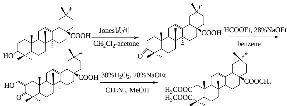
图 2 羊毛甾烷 A 环修饰路线
