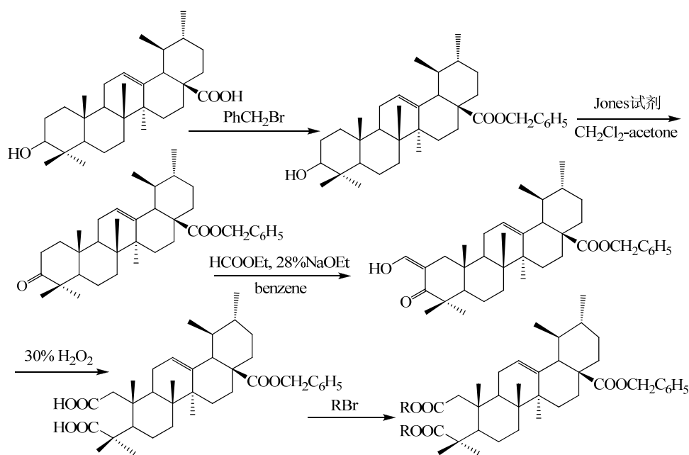
图 4 自行设计的熊果酸 A 环修饰路线
