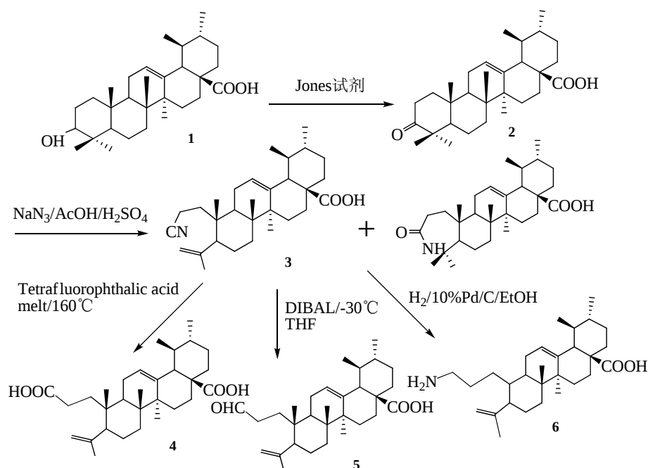
图 3 熊果酸 A 环修饰路线
