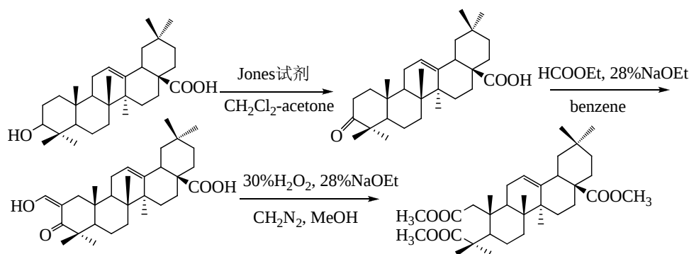
图 1 齐墩果酸 A 环修饰路线
