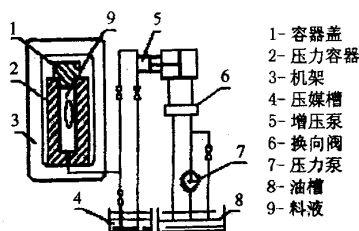
图 2 超高压提取原理示意图
