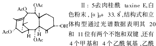
图 2 化合物 II 的结构 II: 5-去肉桂酰 taxine E, 白色粉末, [\alpha]_D^{25} 33.8°, 结构式和立体构型通过光谱数据表明其 20 和 11 位有两个不饱和双键, 还有 4 个甲基和 4 个乙酰氧基, 乙酰化后形成 2 \alpha , 5 \alpha , 9 \alpha , 10 \beta , 13 \alpha -五乙酰氧基-4(20), 11-紫杉二烯(图 2)。
