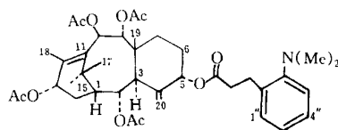
图 1 化合物 I 的结构
