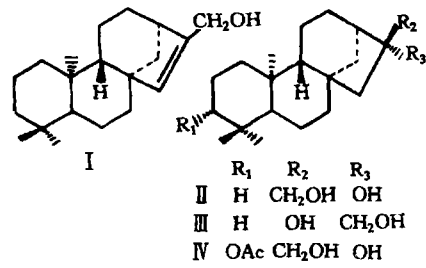
图 1 化合物Ⅰ~Ⅳ的化学结构式
