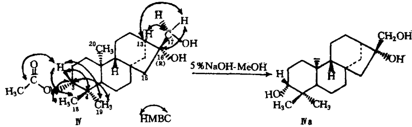
图 2 Ⅳ和Ⅳa 的 HMBC 分析
