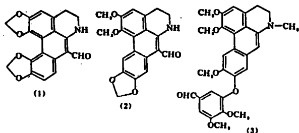
图 莲叶桐中新阿扑啡生物碱的结构
