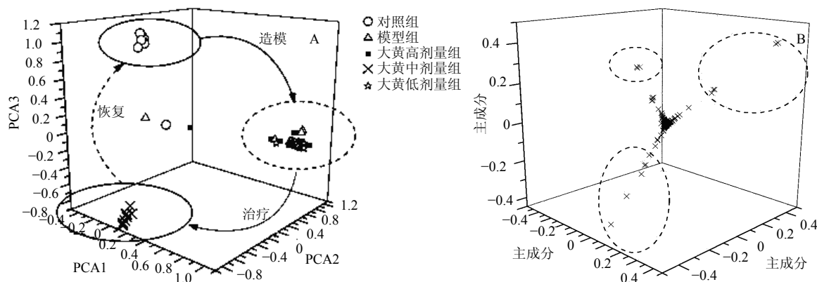
图2 大黄水煎液给药后各组大鼠尿液代谢产物得分图(A)和荷载图(B)
